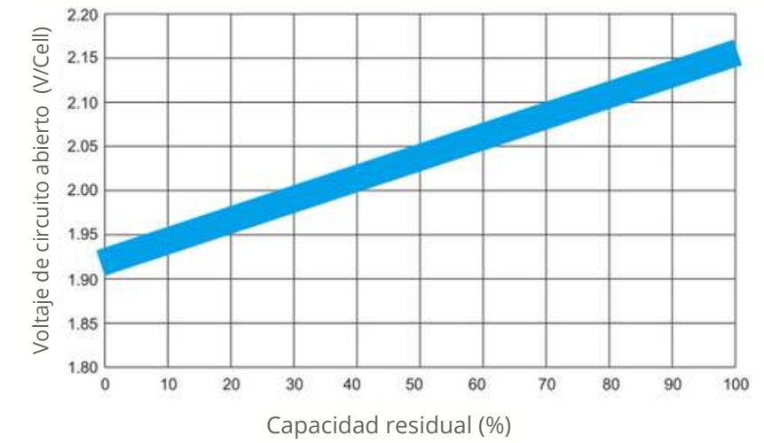
Voltaje de circuito abierto VS Capacidad residual
